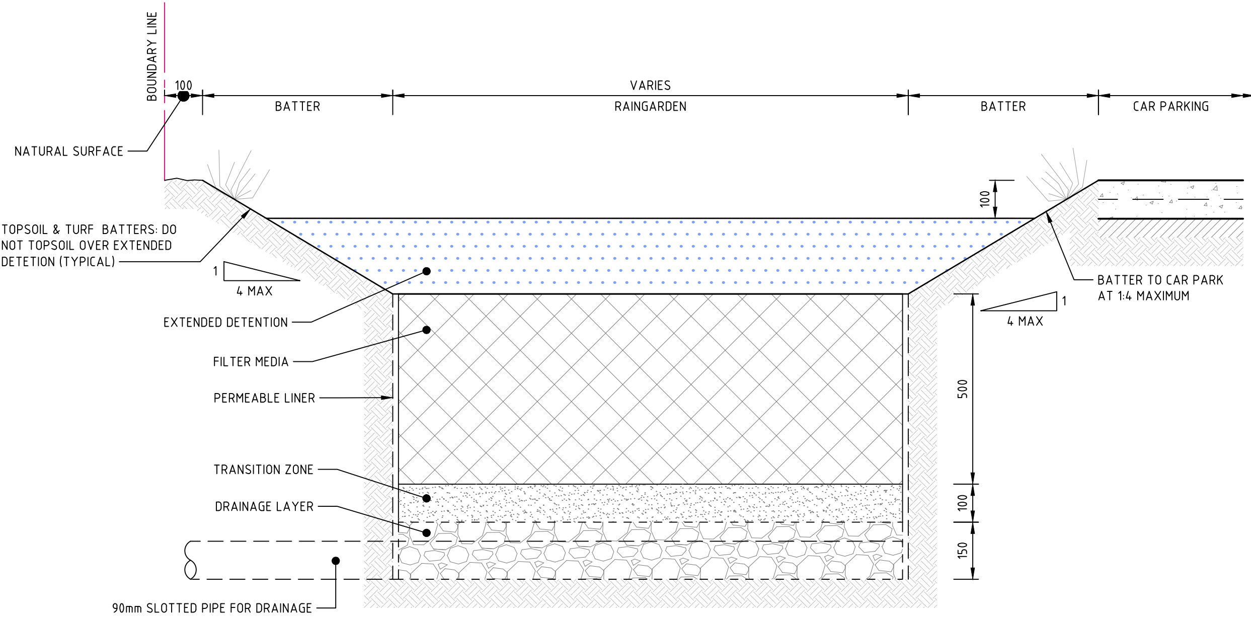
SECTION A SCALE 1:10 C03
